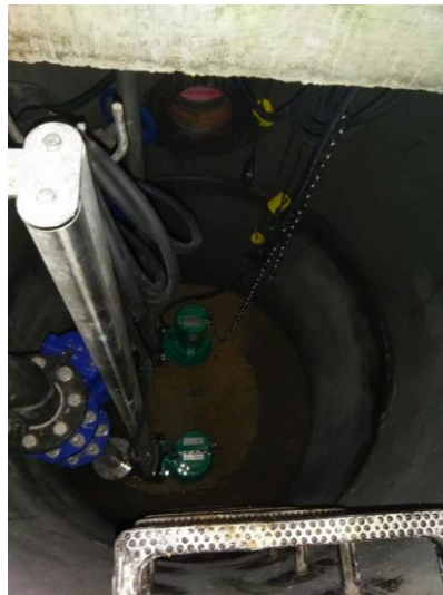
CSÁ-3 csapadékáttemelő
